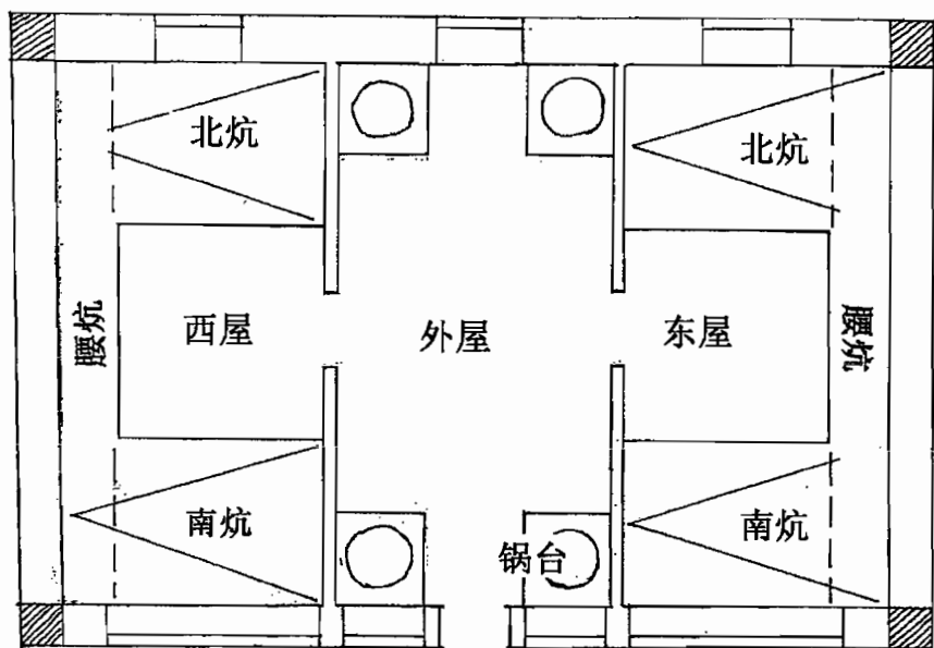
图一 传统南北炕格局
